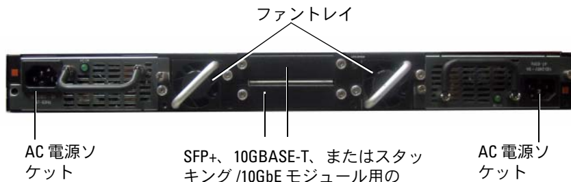
図 1-10. PC7048R の背面パネル
